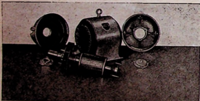
Afbeelding 1. Uit elkaar genomen S.K.A.-motor 15 pk, 1450 omw/min.
