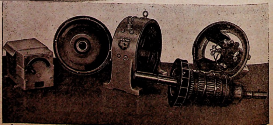
Afbeelding 3. Uit elkaar genomen gelijkstroommotor 15 pk, 1450 omw/min. met aanloopweerstand.
